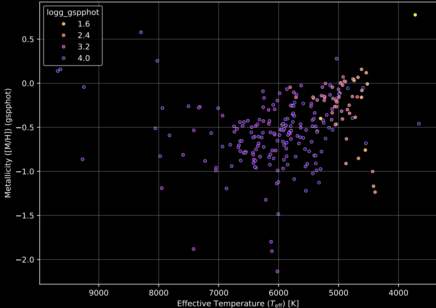
GALAH DR4 Field: [3886] Stellar Population Parameters (n= 238)
