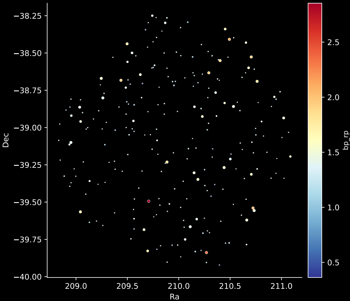
GALAH DR4 Field: [3886] Stars: 238
