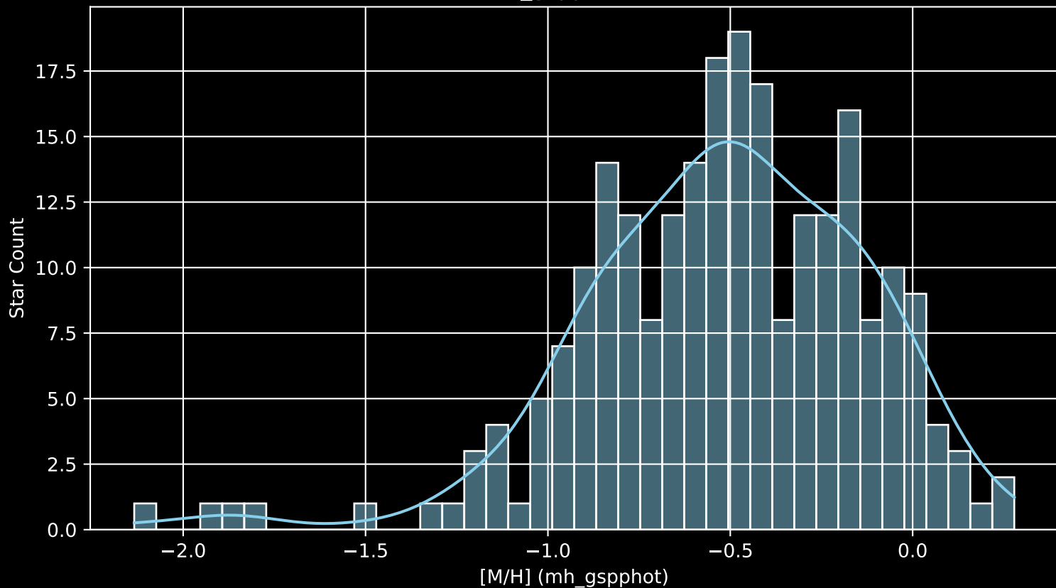
GALAH DR4 Field: [3886] [M/H] (mh_gspphot) (n= 236)
