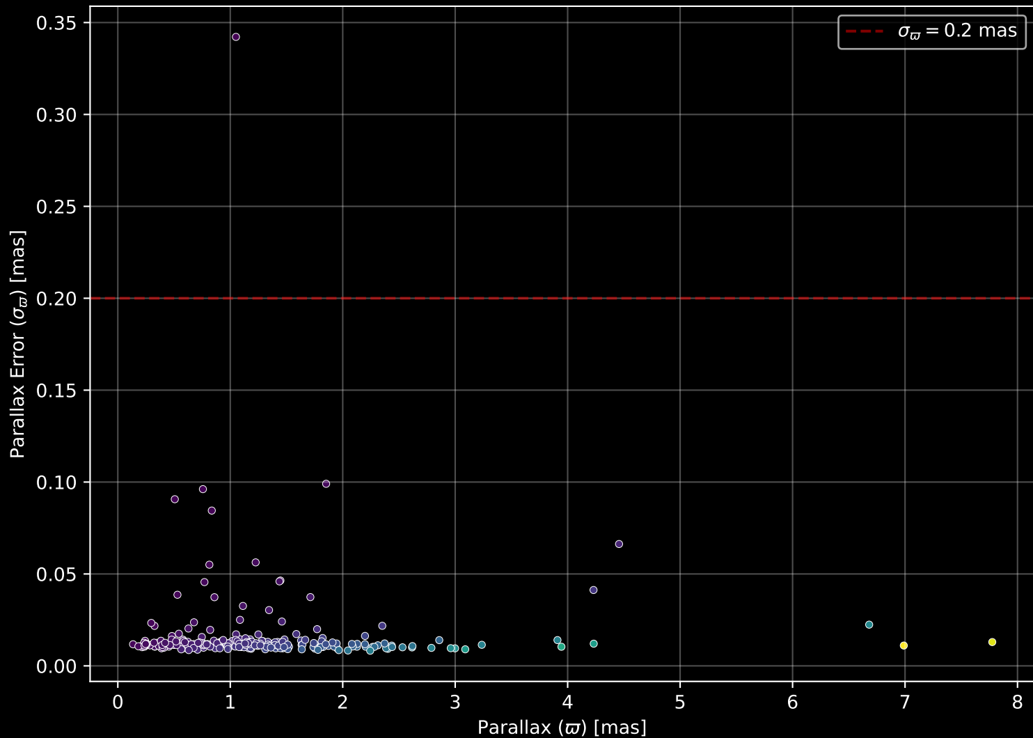
GALAH DR4 Field: [3886] Parallax Quality (n= 238)
